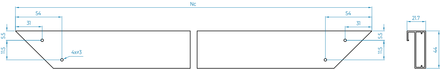
DT22110: KHUNG CÁCH TỦ SL: 2
