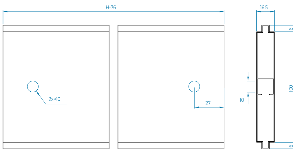
DT22123: LÁ PHẪNG 16.5MM 2 ĐẦU
