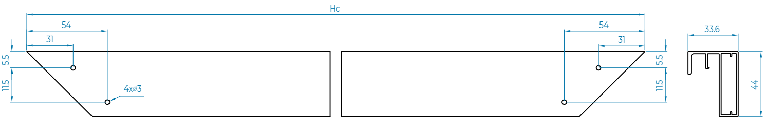
DT22110: KHUNG CÁCH TỦ MỞ SL: 1
