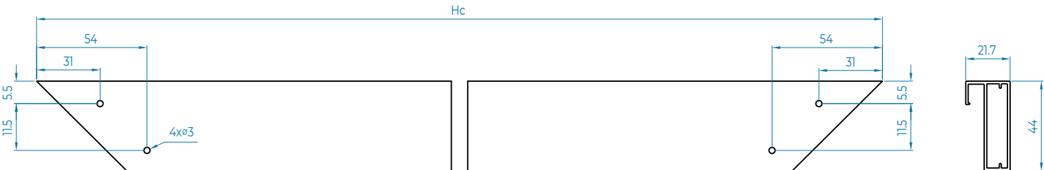
DT22110: KHUNG CÁCH TỦ SL: 1
