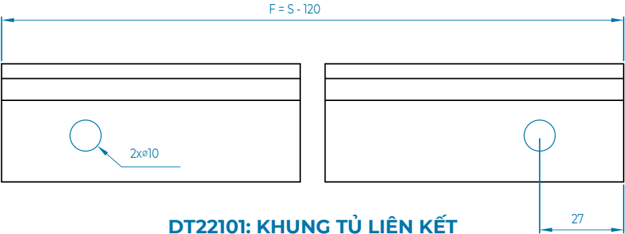
DT22101: KHUNG TỦ LIÊN KẾT DẬP LỖ Ø102 ĐẦU
