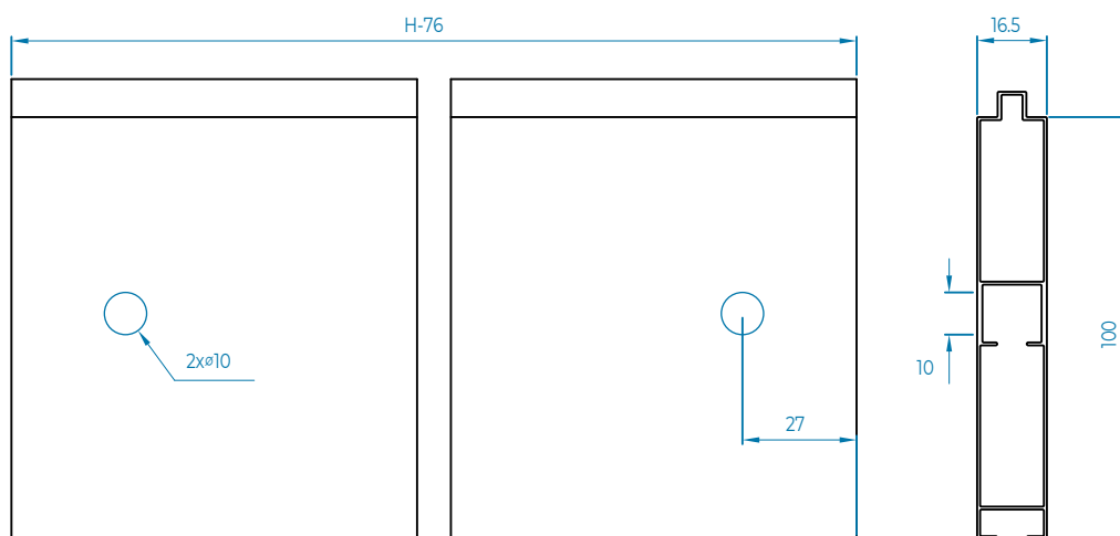
DT22122: LÁ PHẪNG 16.5MM 1 ĐẦU
