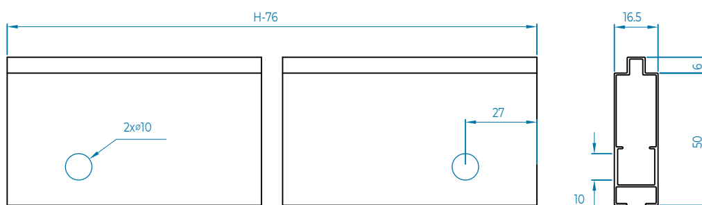
DT22124: LÁ PHẪNG 16.5MM NHỎ
